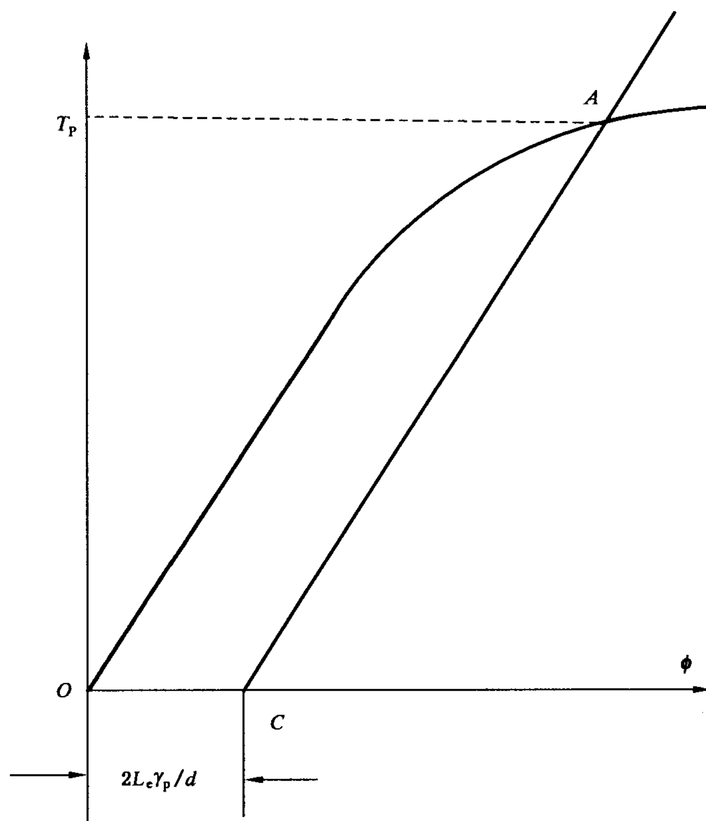
图 4 规定非比例扭转强度
