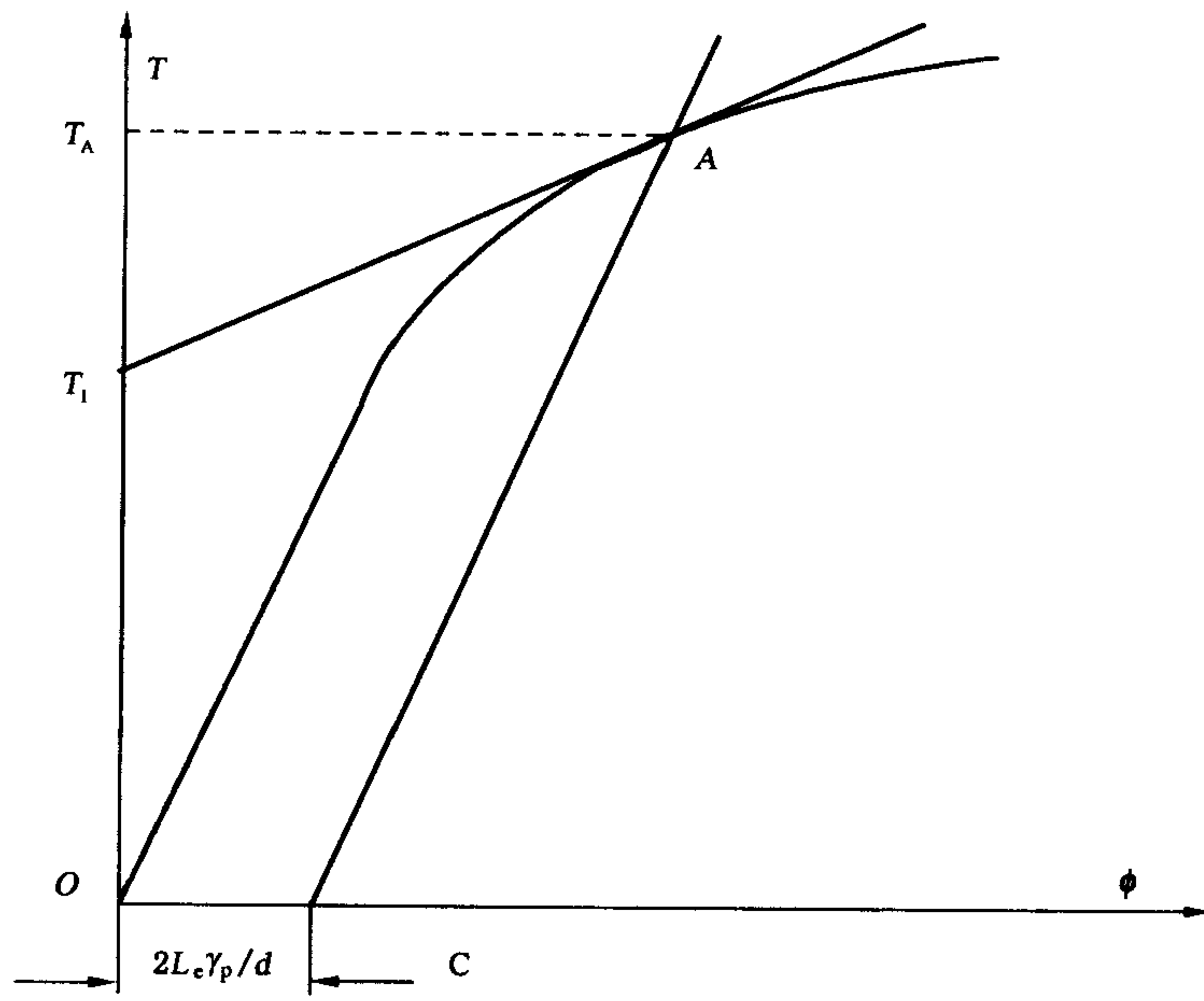
图 B.1 真实规定非比例扭转强度
