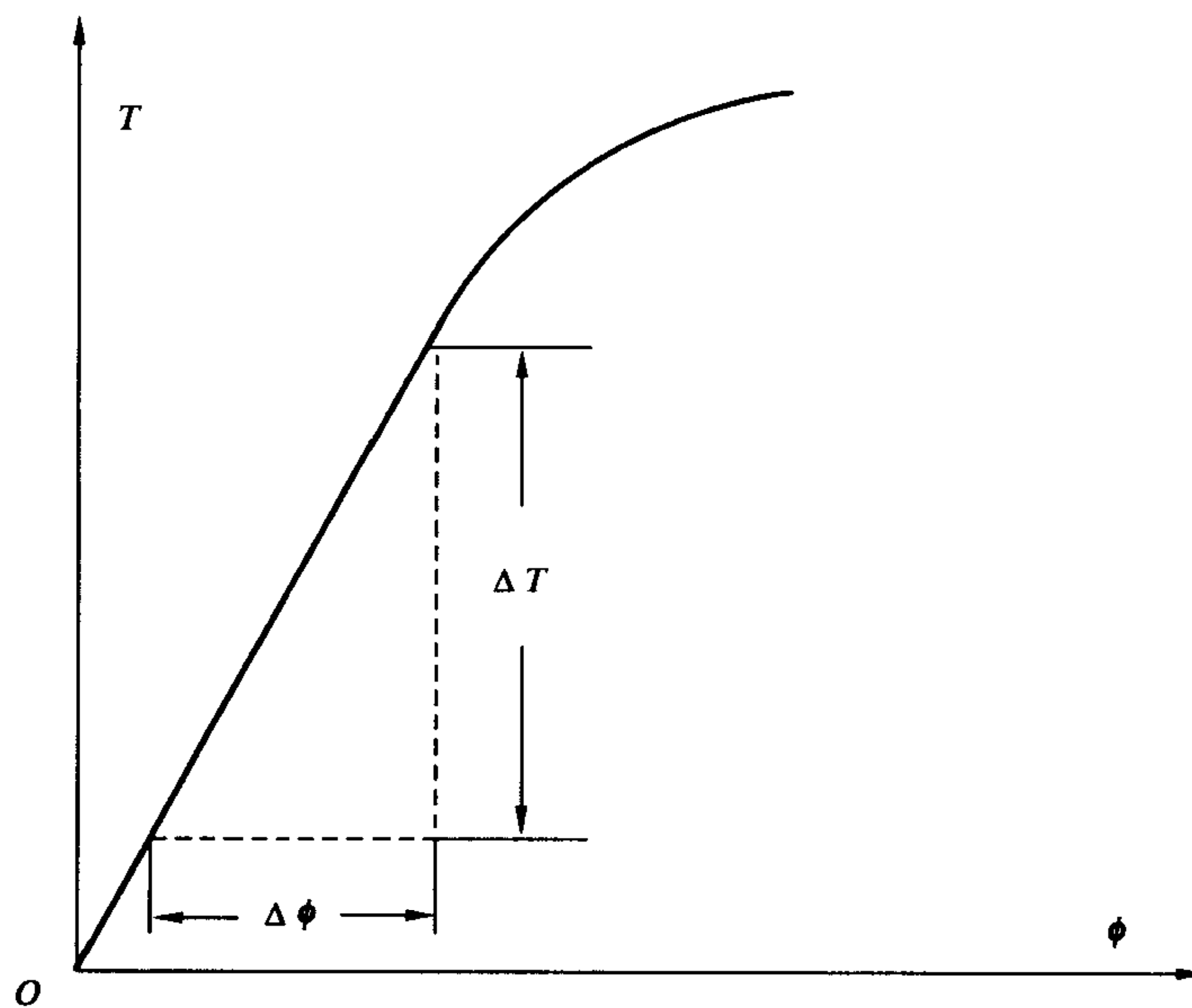
图 3 剪切模量
