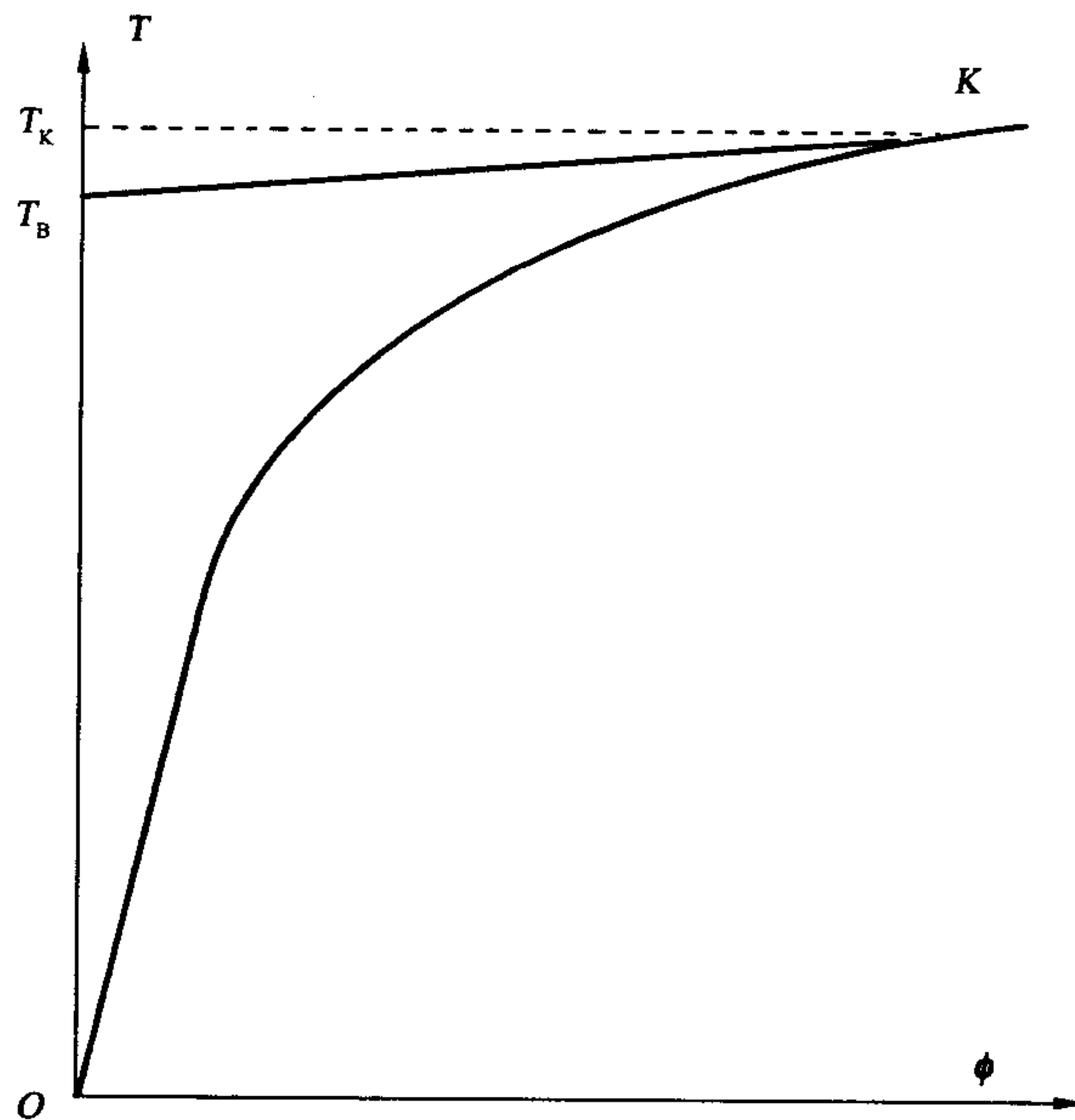
图 B.2 真实抗扭强度
