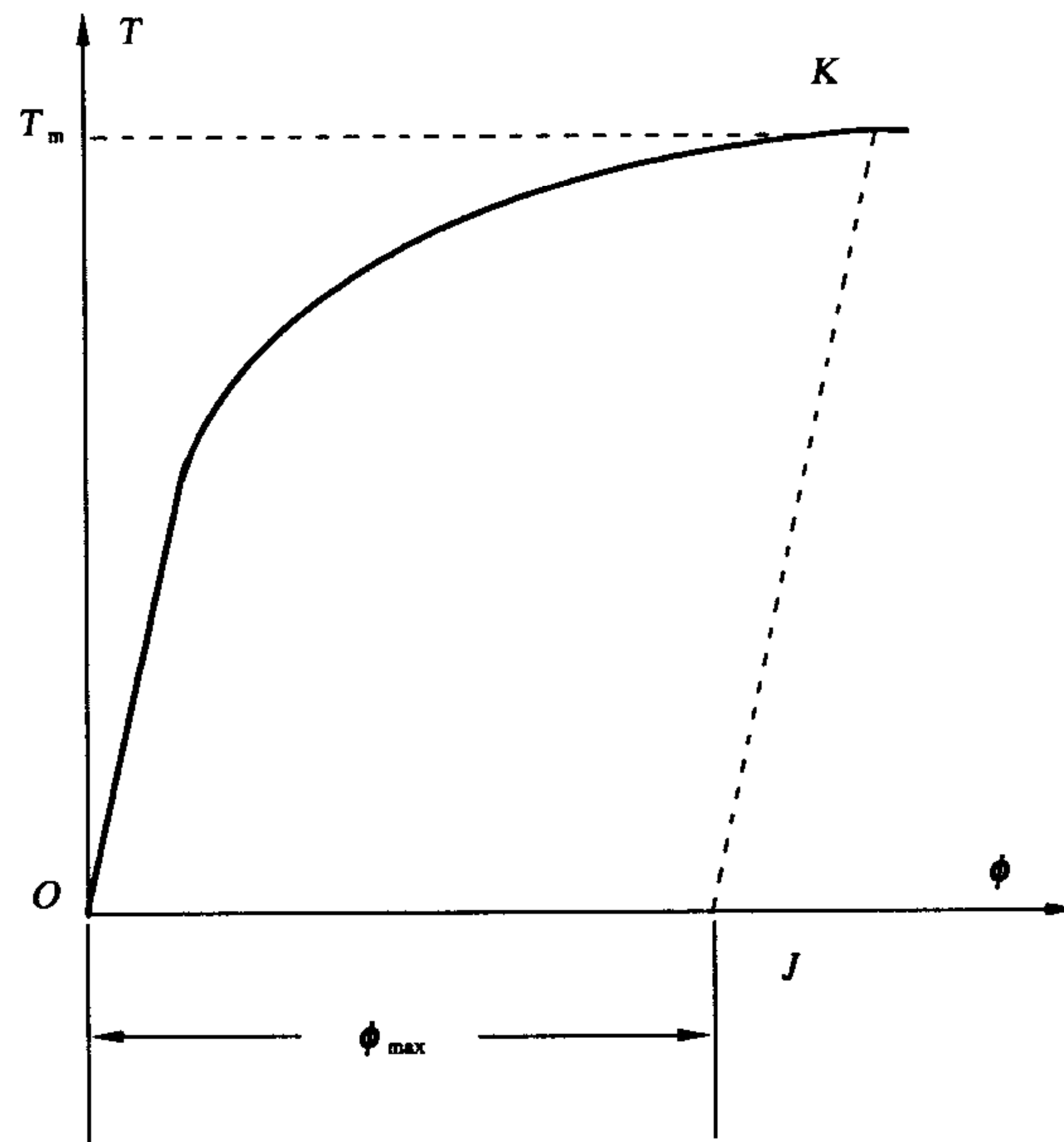
图6 抗扭强度
