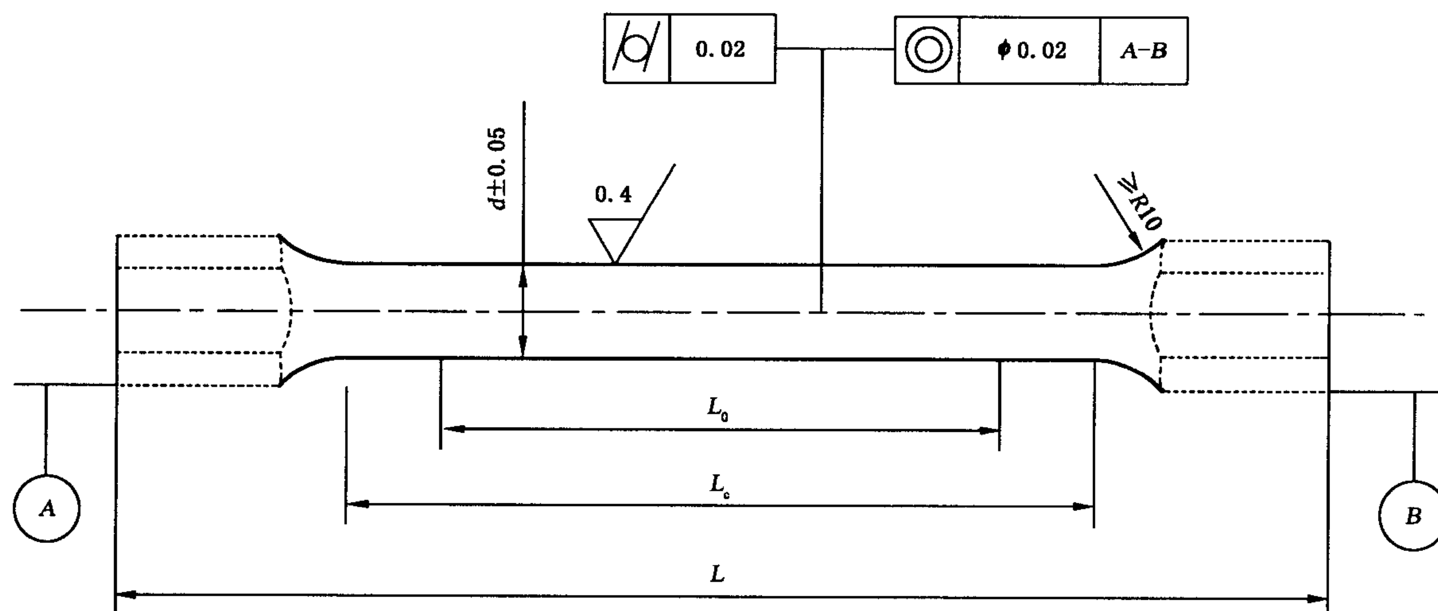
图 1 圆柱形试样
